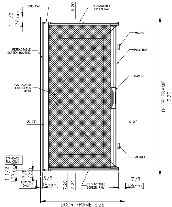
INSWING DOOR OUTSWING DOOR
