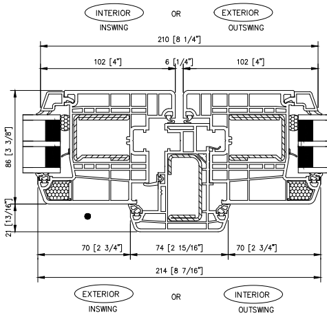
12 4700 - JAMB
