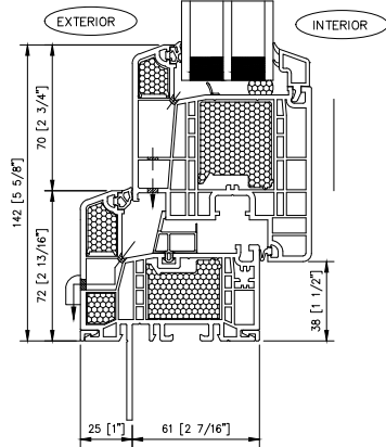
2 4700 INSWING - SILL
