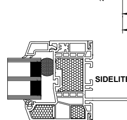
11 4700 - JAMB
