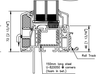
8 4700 SIDELITE - SILL
