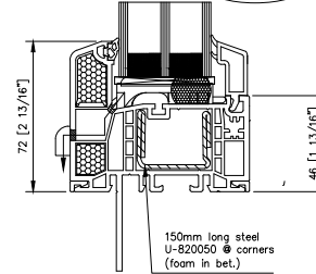
4 4700 SIDELITE - SILL
