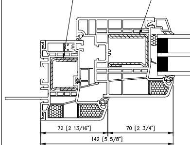
9 4700 - JAMB
