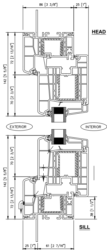
2 4700 INSWING - SILL
