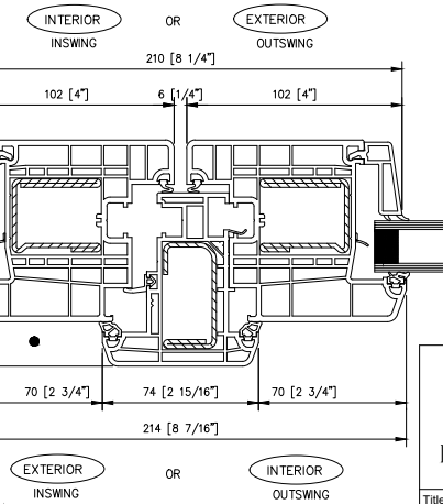
12 4700 - JAMB
