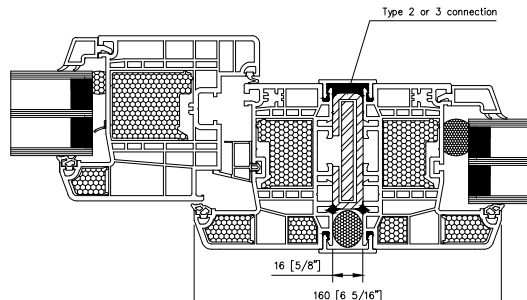
10 4700 - JAMB
